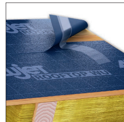
► Fixierung der Bahn mit dem integrierten Klebestreifen
