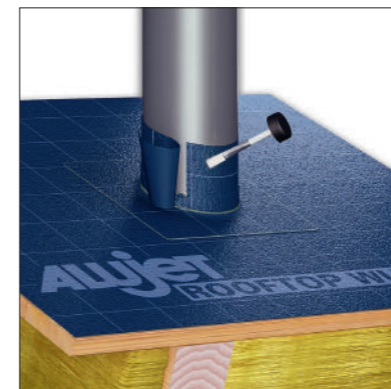
► Ausführung wasserundurchlässige Verklebung Dunstrohdurchgang
