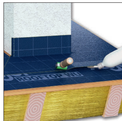
► Ausführung / Verschweißung aufgehendes Bauteil
