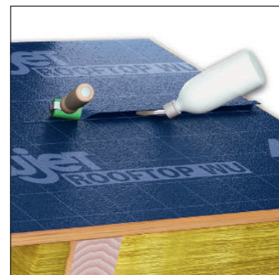
► Ausführung wasserundurchlässige Verschweißung der Überlappung
